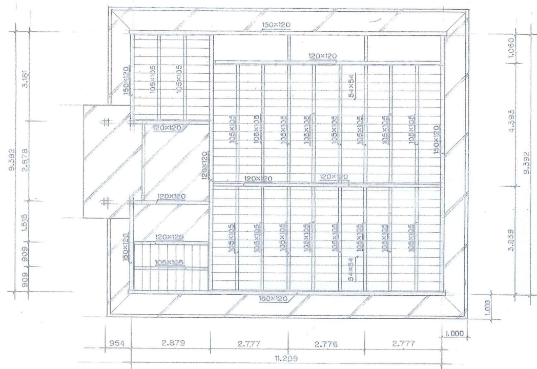
一階床伏図 S=1/100
