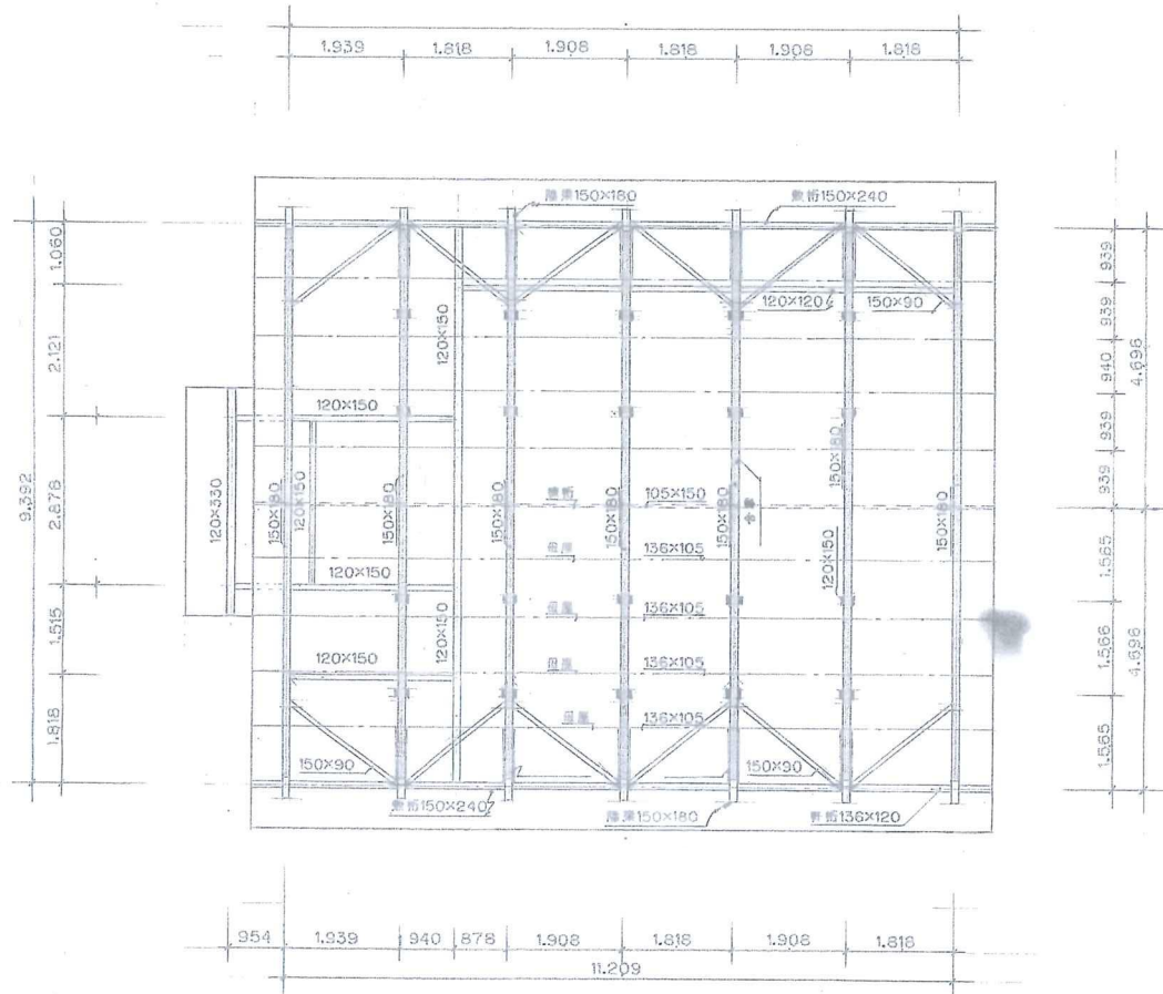
二階床伏図 S=1/100
