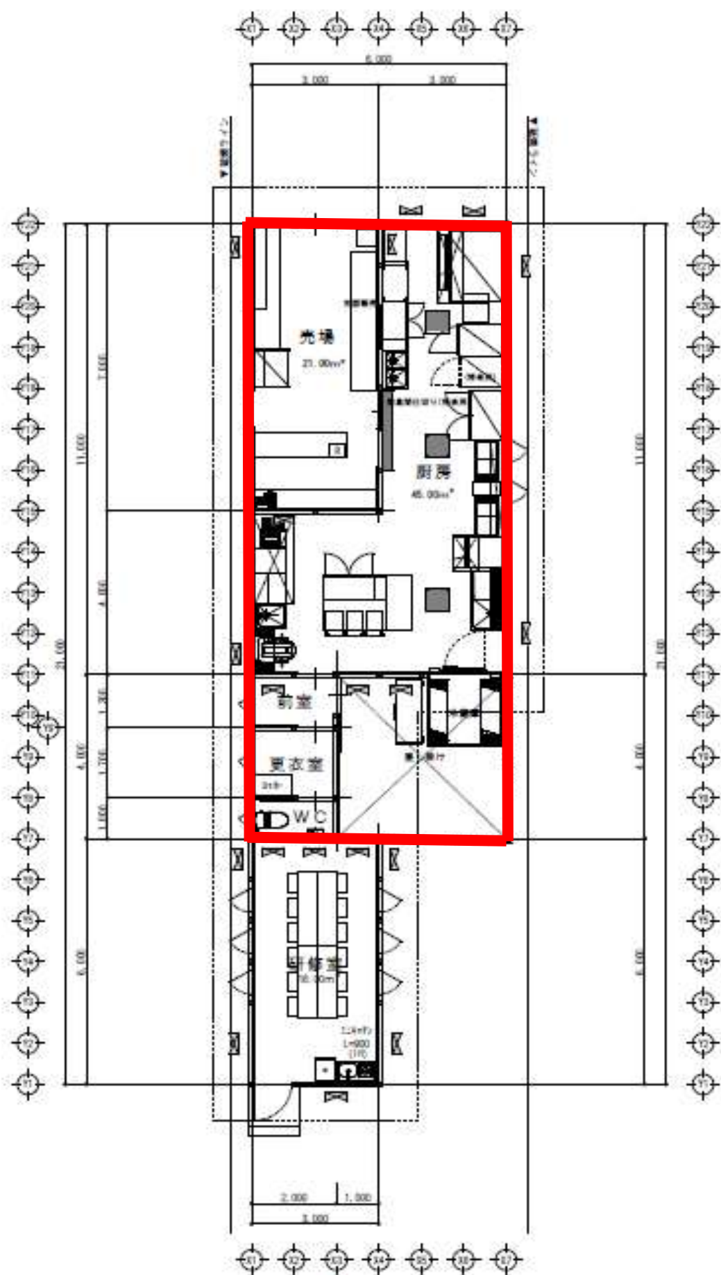
平面図 S:1/100
